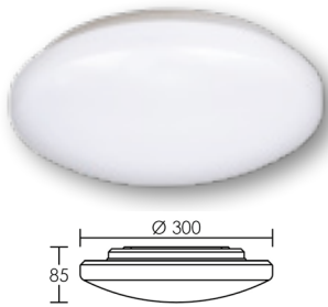
Version 16W sans anneau
