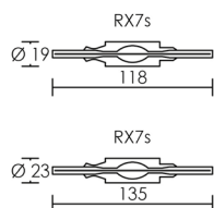
Lampe iodures brûleur quartz. Culot RX7s.
