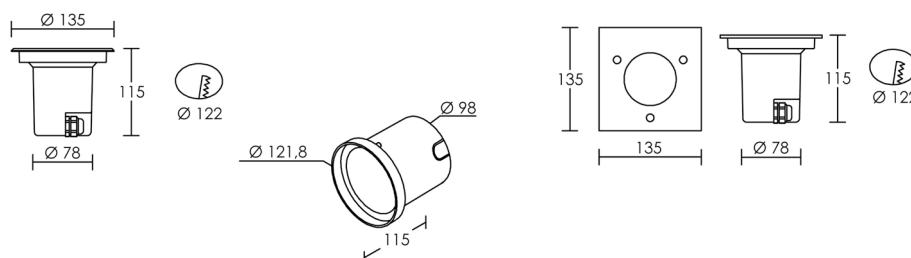
Boîte d'encastrement commune aux 2 modèles
